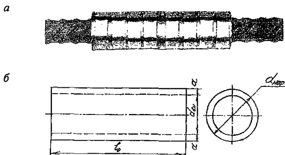
Рисунок В.1: a – опрессованный стык построечного изготовления, произведенный на мобильном оборудовании многократным поперечным деформированием соединительной муфты с промежутками, б – соединительная муфта для опрессованных стыков
