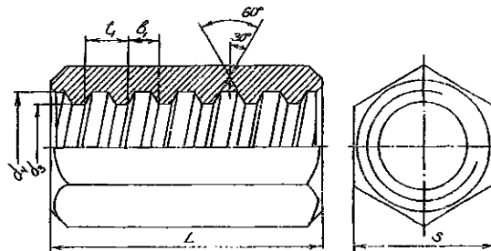
Рисунок В.3 - Резьба соединительных элементов для арматуры винтового профиля.
